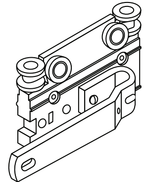
Baton Master Carrier - R.H. 8400-10
